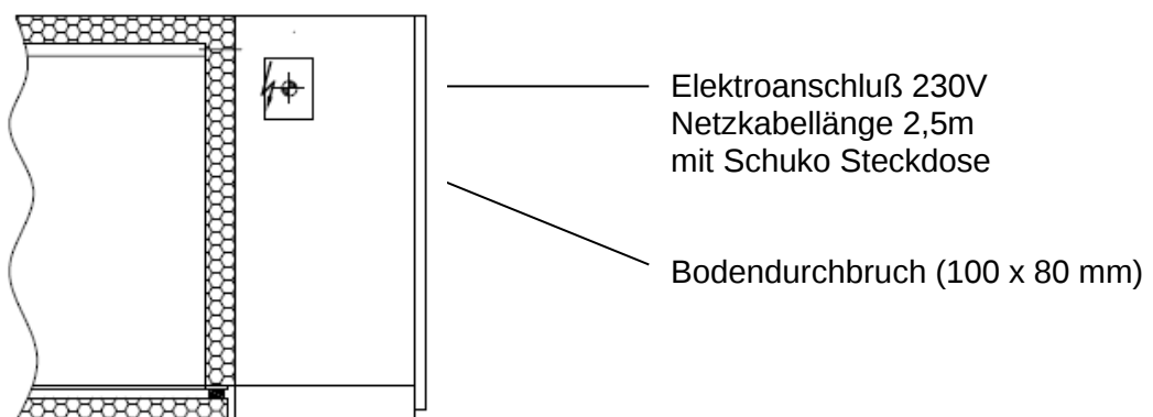
Bild 3: Draufsicht Kühltisch (Eigenkühlung, steckerfertig)
